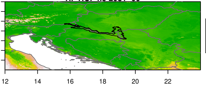
RF RCP4.5 2081-00
