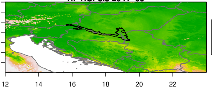
RF RCP8.5 2041-60
