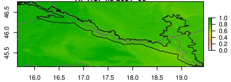
RF RCP4.5 2081-00
