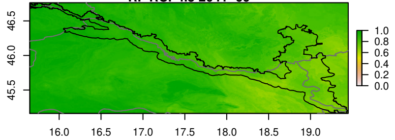
RF RCP4.5 2041-60
