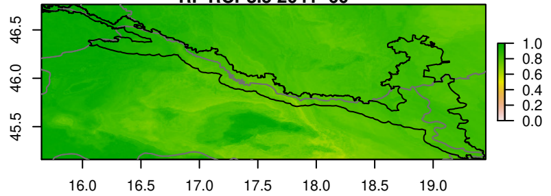
RF RCP8.5 2041-60
