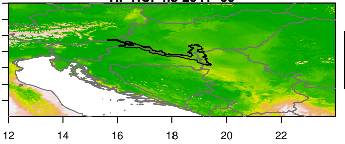
RF RCP4.5 2041-60
